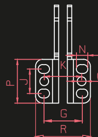
Model: 1101 A-L
