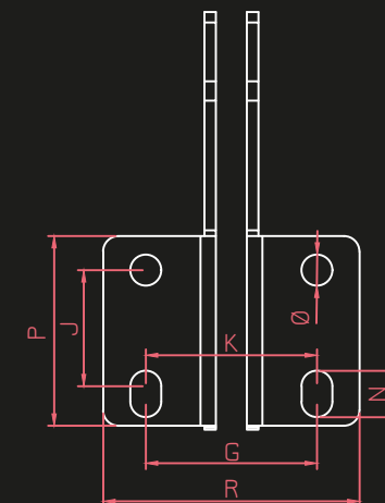
Model: 1104 A-L
